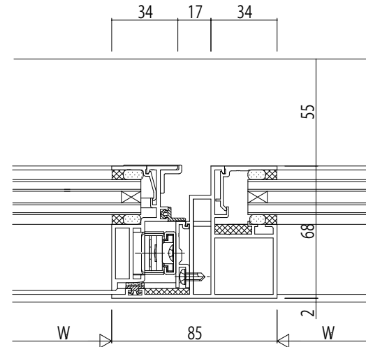
たて骨部(すべり出し+F I X)
