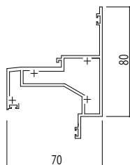
●外倒し窓・突出し窓(隠ぺい)/ピボットヒンジドア
