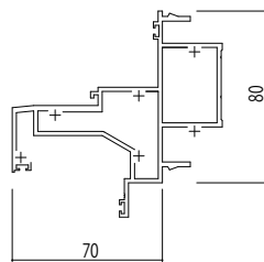
●外倒し窓・突出し窓(隠ぺい)/ピボットヒンジドア高強度無目仕様
