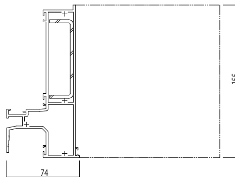
●FIX窓/自動ドア(上かまち隠ぺい)
