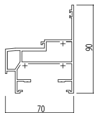
●外倒し窓・突出し窓(隠ぺい)/フロアヒンジドア
