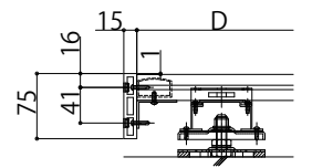
デッキ高さ:85~100mmの場合
