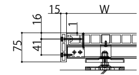
デッキ高さ:85~100mmの場合
