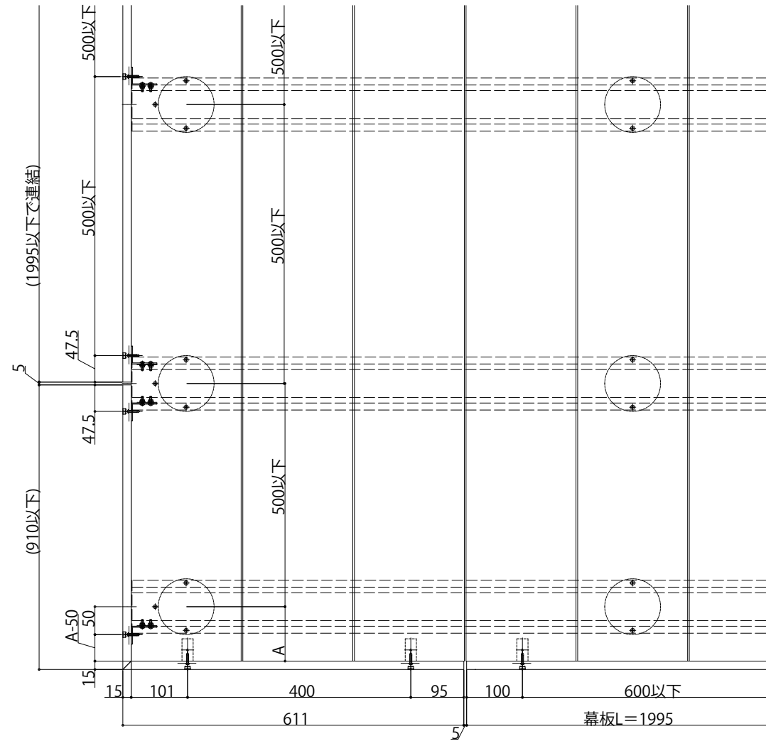
幕板連結部
