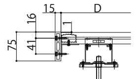
デッキ高さ:130~160mmの場合
