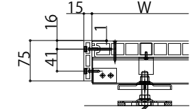
デッキ高さ:100~130mmの場合
