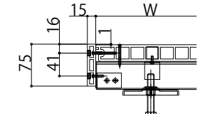
デッキ高さ:130~160mmの場合
