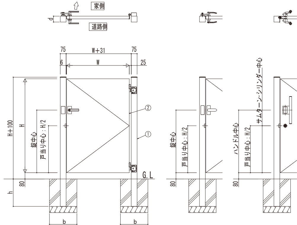
打掛錠1型の場合
