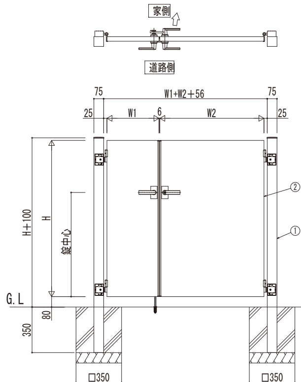
打掛錠1型の場合
