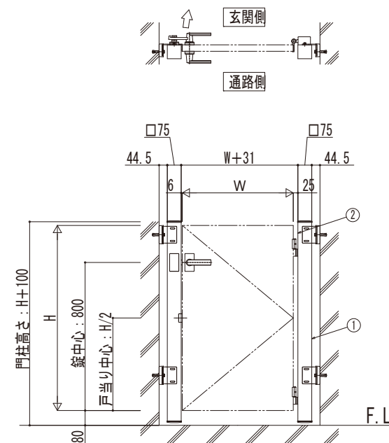
調整用スペーサー有りの場合
