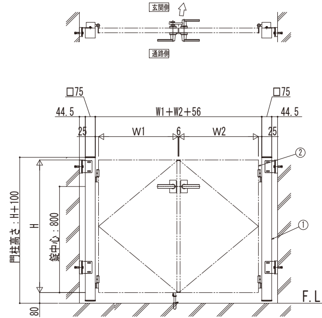
調整用スペーサー有りの場合
