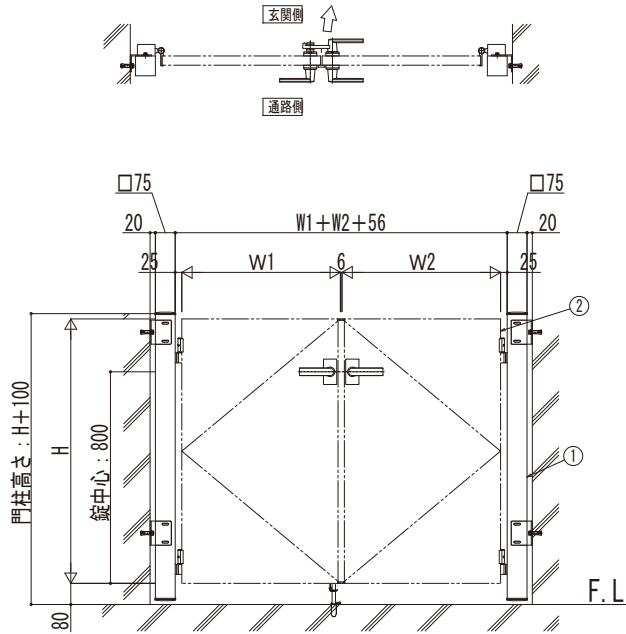
調整用スペーサー無しの場合
