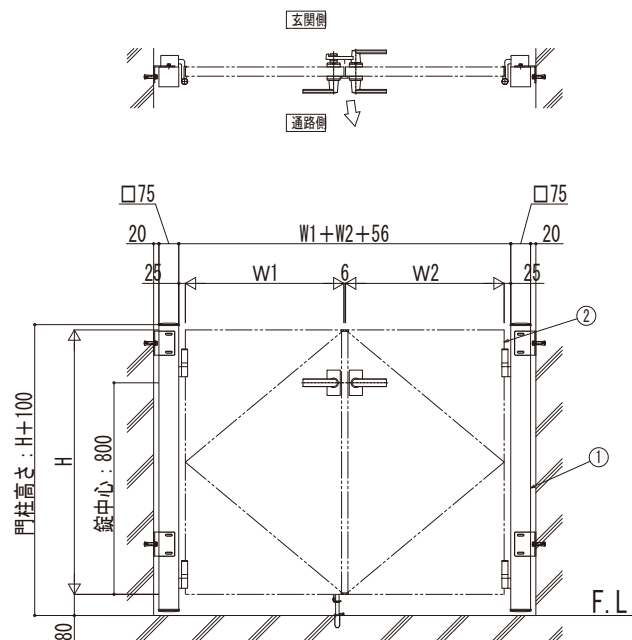
調整用スペーサー無しの場合
