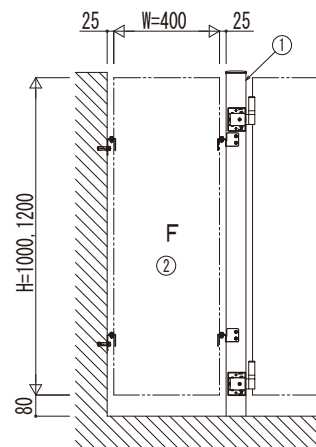
壁-門柱納まり 外開き
