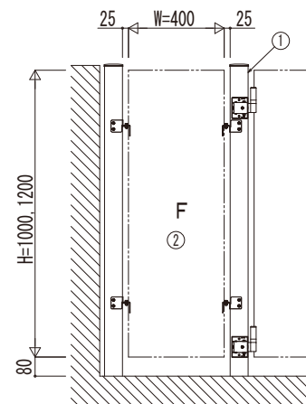
門柱-門柱納まり 外開き
