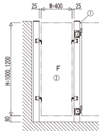
門柱-門柱納まり 内開き
