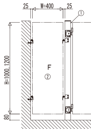
壁-門柱納まり 内開き
