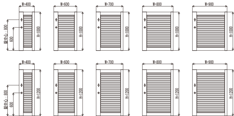
レバーハンドル・プッシュプル仕様の場合
