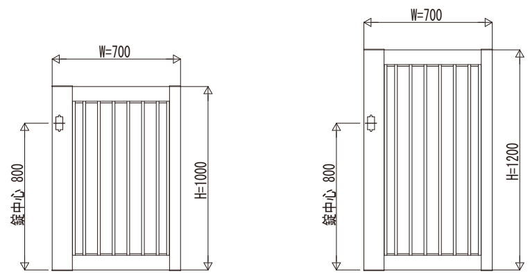
打掛錠仕様の場合
