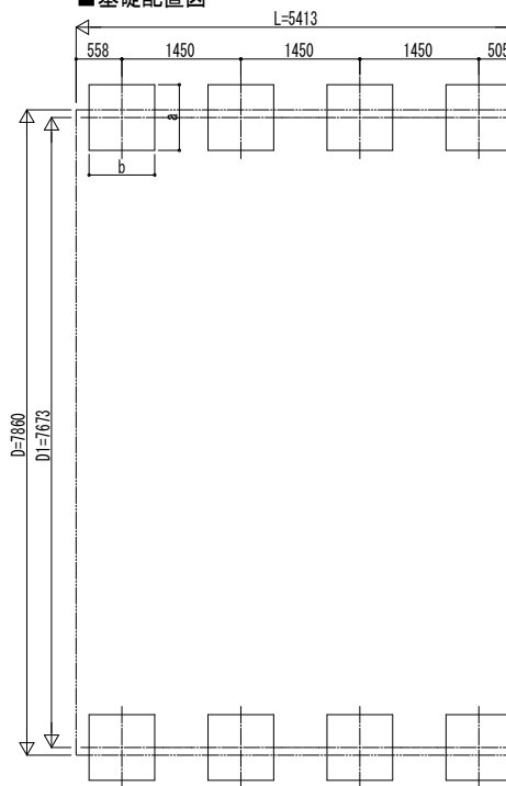
■ 基礎配置図
