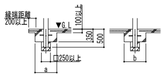
■ 姿図 土間コンクリート同時施工基礎の場合
