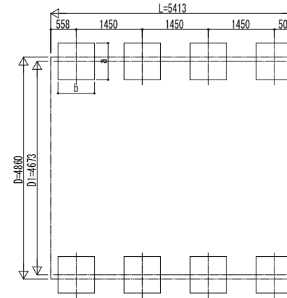
■ 基礎配置図
