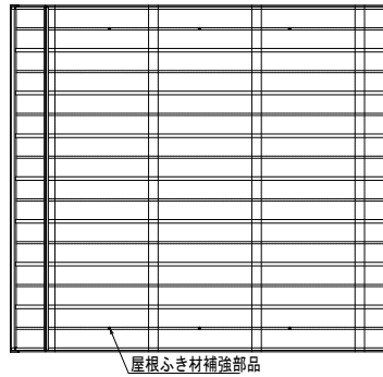
■ 姿図
