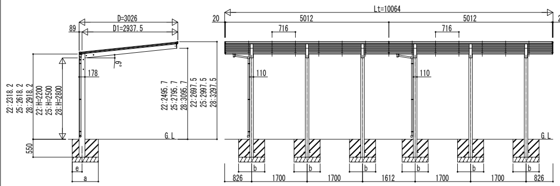
独立基礎の場合
