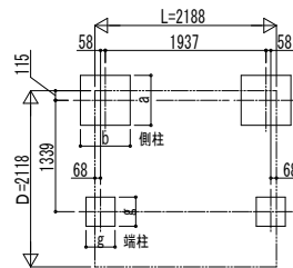
■ 基礎配置図
