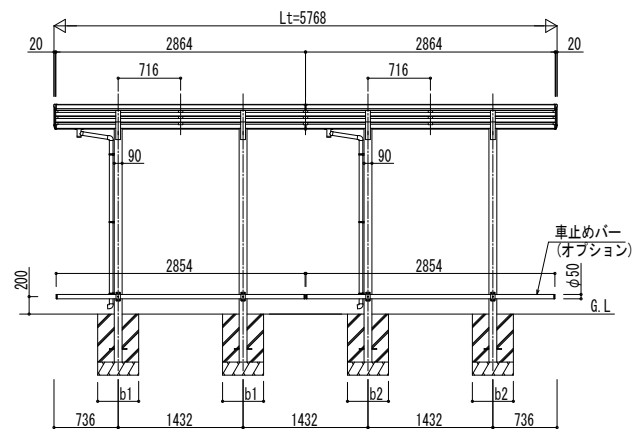
■ 基礎寸法表
