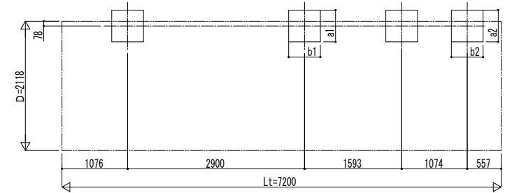
■ 基礎配置図
