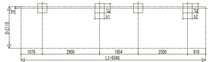
■ 基礎配置図
