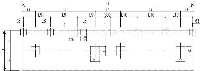
■基礎配置図
