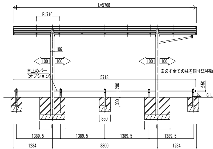
■ 基礎寸法表
