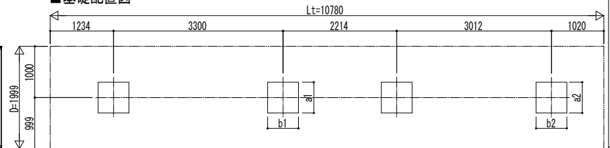
■ 基礎配置図
