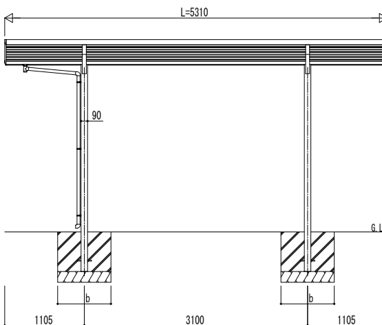
■基礎寸法表
