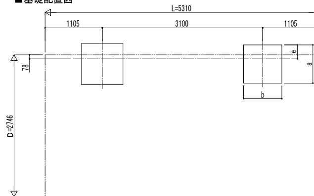
■基礎配置図
