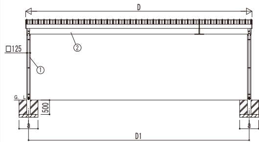
■基礎断面図 独立基礎の場合
