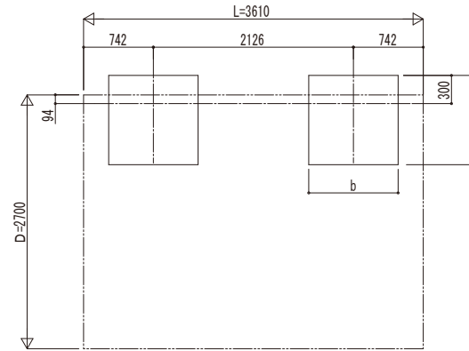
■ 基礎配置図
