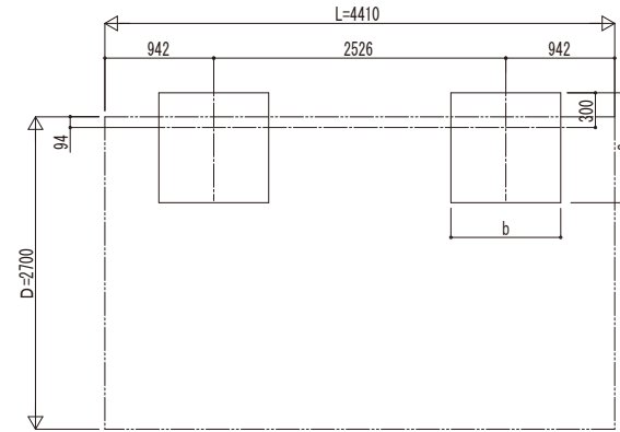
■ 基礎配置図
