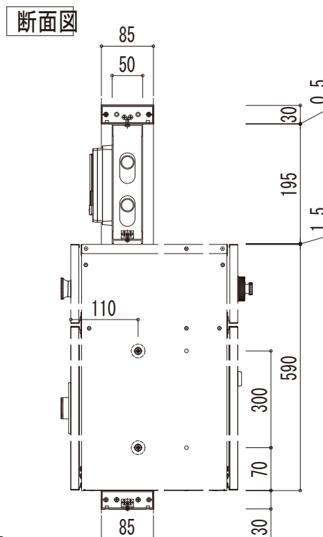
B-B断面図
