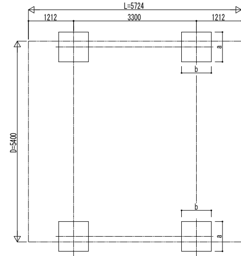
■ 基礎配置図
