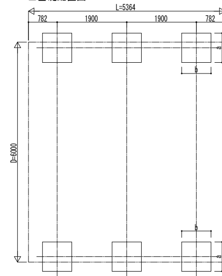
■ 基礎配置図
