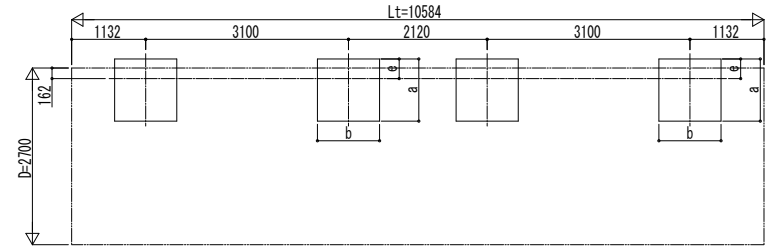
■ 基礎配置図
