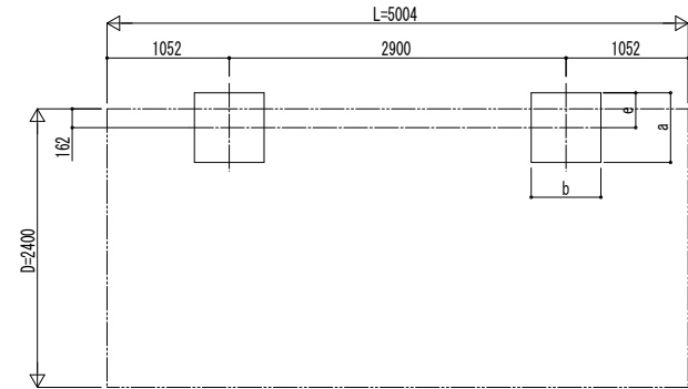
■基礎配置図
