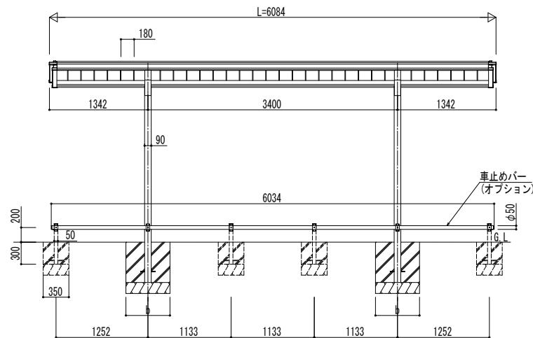
■ 基礎寸法表
