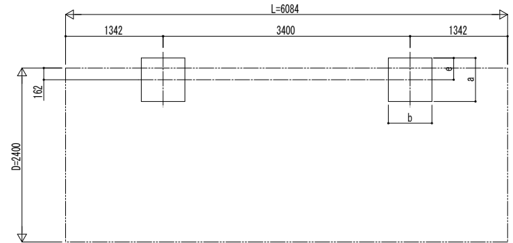
■ 基礎配置図
