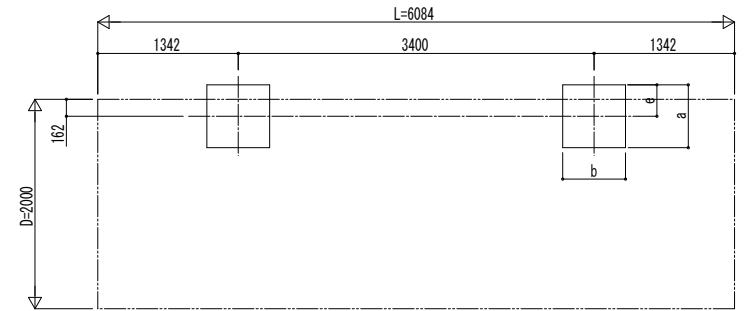
■ 基礎配置図
