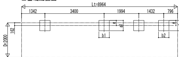
■ 基礎配置図
