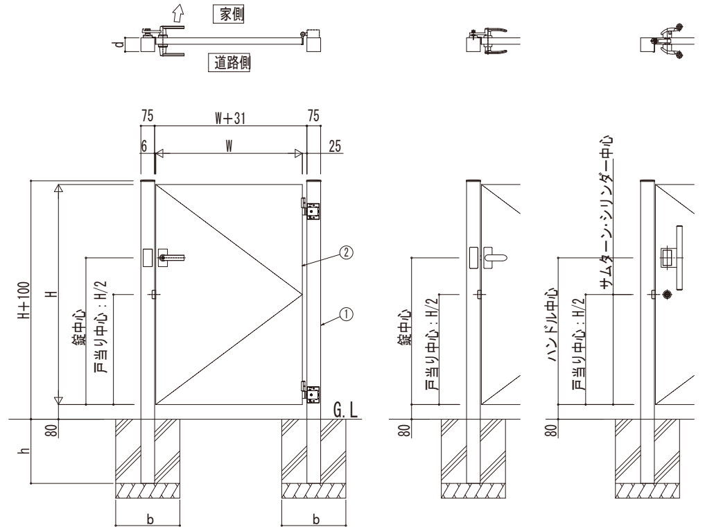
打掛錠1型の場合
