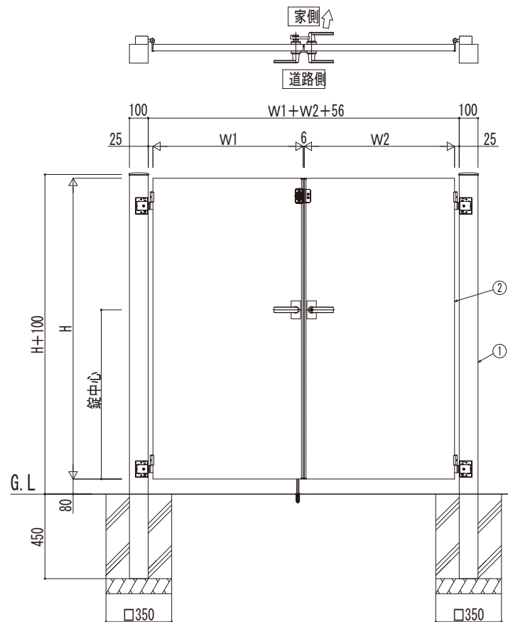
打掛錠1型の場合
