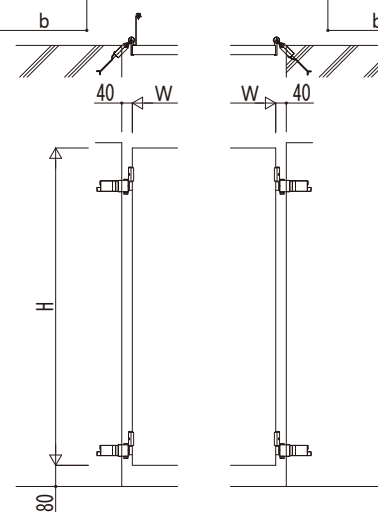
埋込金具納まり 吊元部
