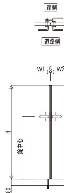
打掛錠2型の場合
