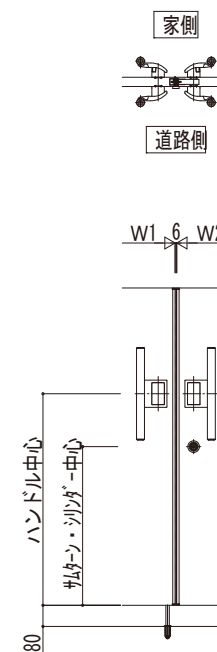
ラッチ錠の場合
