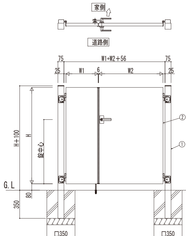
打掛錠I型の場合
