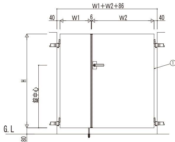
打掛錠1型の場合
