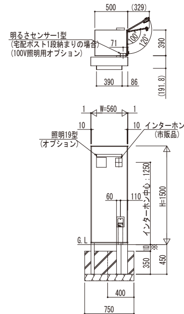
1段納まりの場合
