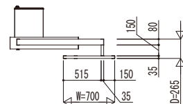
ルシアスウォールHJ01型 +プリードウォールフレームユニットN02型
