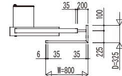
ルシアスウォールHJ01型 +プリードウォールフレームユニットN03型
