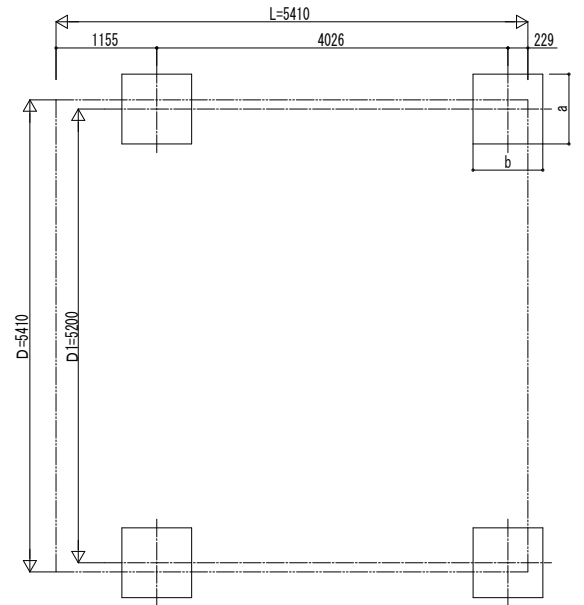
■基礎配置図
