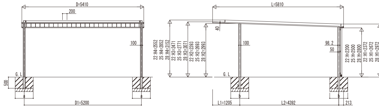
独立基礎の場合
