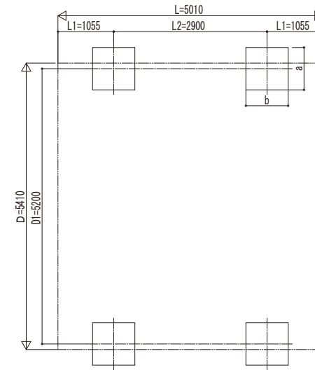
■ 基礎配置図
