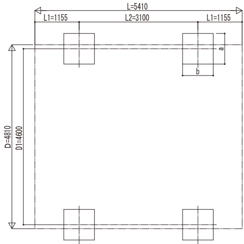
■ 基礎配置図
