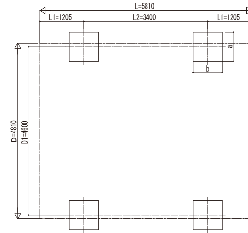
■ 基礎配置図
