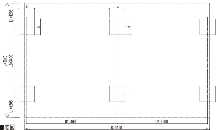
■基礎配置図
