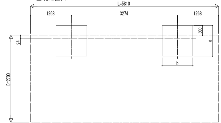
■ 基礎配置図
