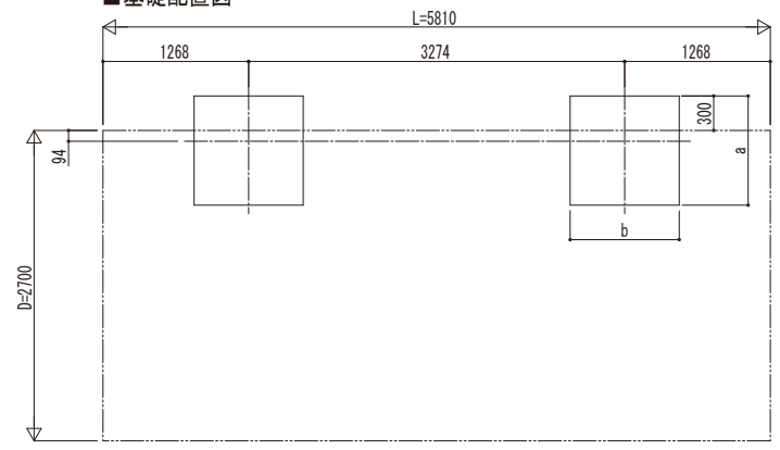
■ 基礎配置図
