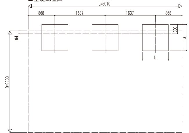
■基礎配置図
