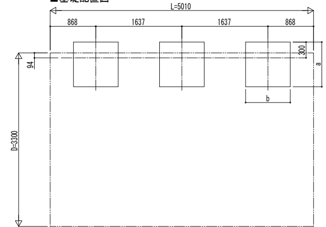
■ 基礎配置図
