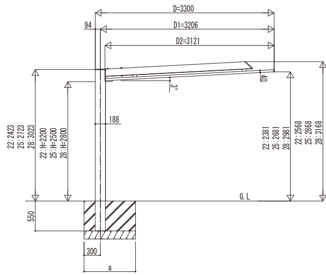
独立基礎の場合
