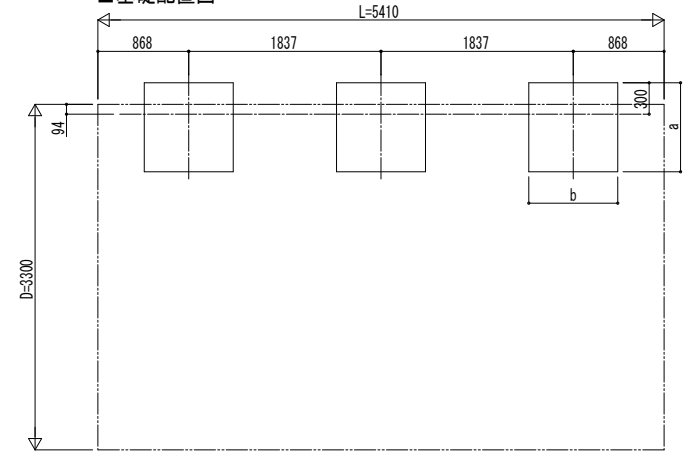
■ 基礎配置図
